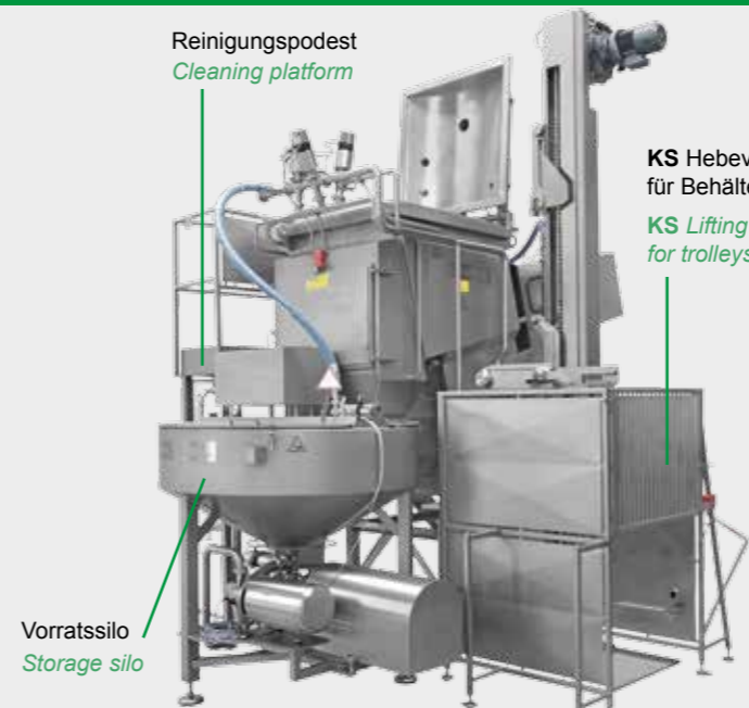
▼ KS Mischer 400 Typ 770 KS Mixer 400 Type 770
